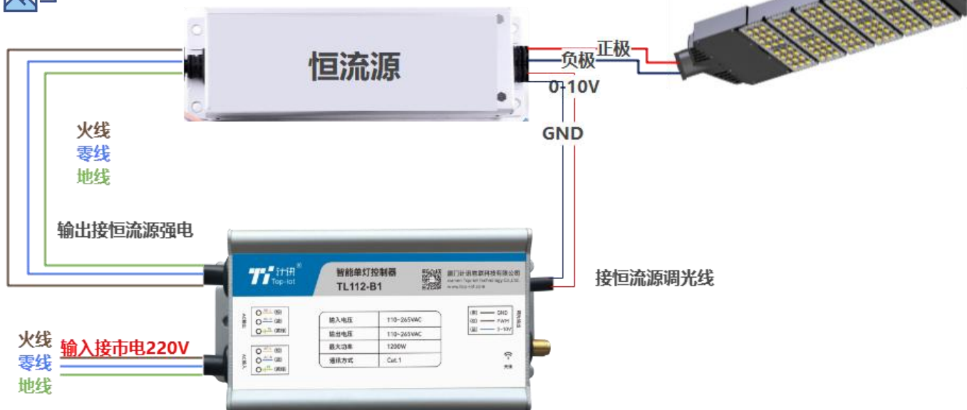
接线示意图
